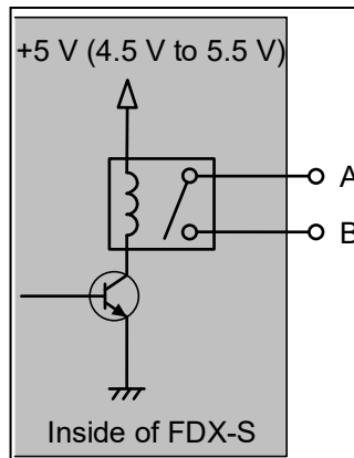
[Fig. 10.47] Alarm output
