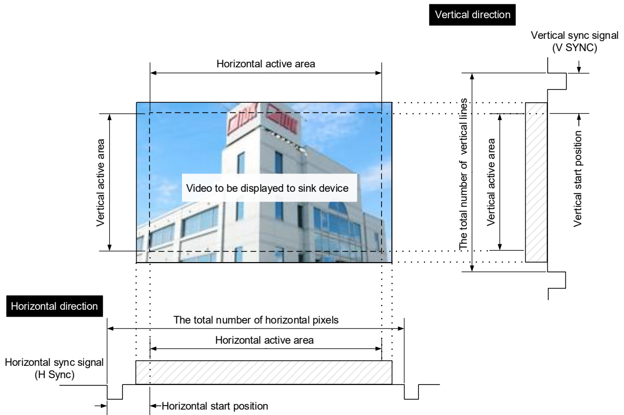
[Fig. 10.21] Input area
