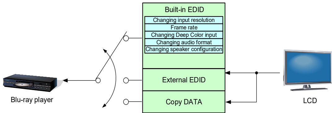
[Fig. 10.23] Setting EDID
