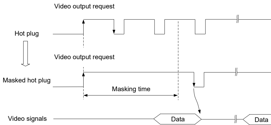
[Fig. 10.17] Hot plug mask
