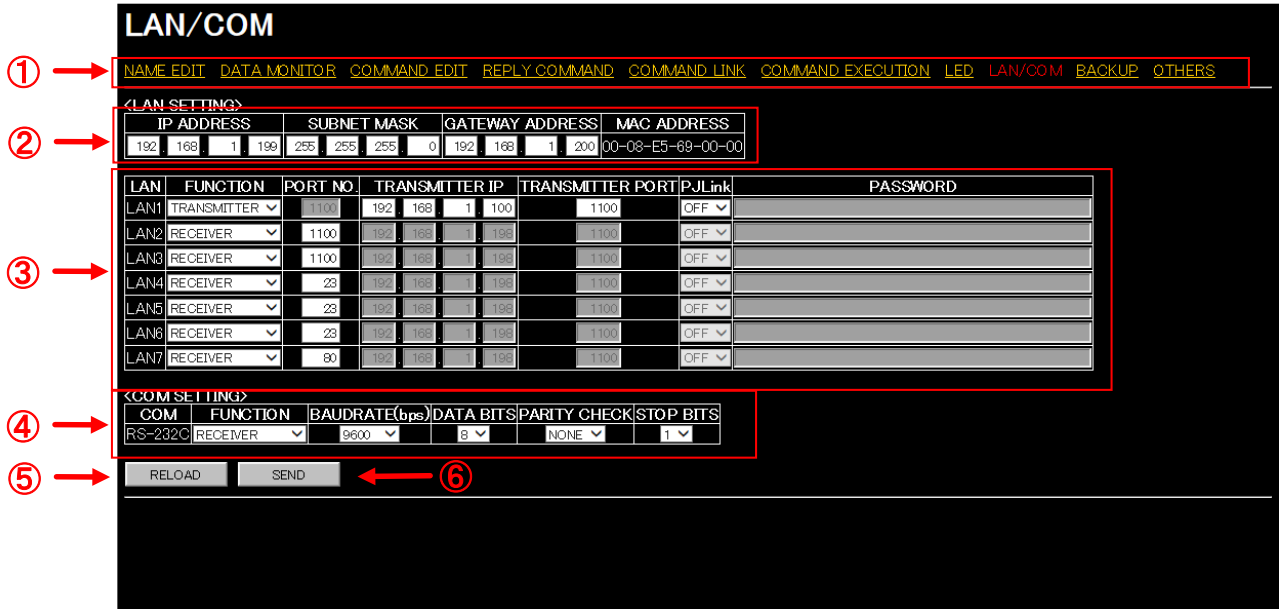
[Fig. 9.38] LAN / COM menu
